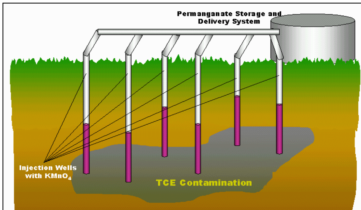
Abbildung 5: Prinzipskizze zur In-situ-chemischen-Oxidation (Quelle: US-EPA)
