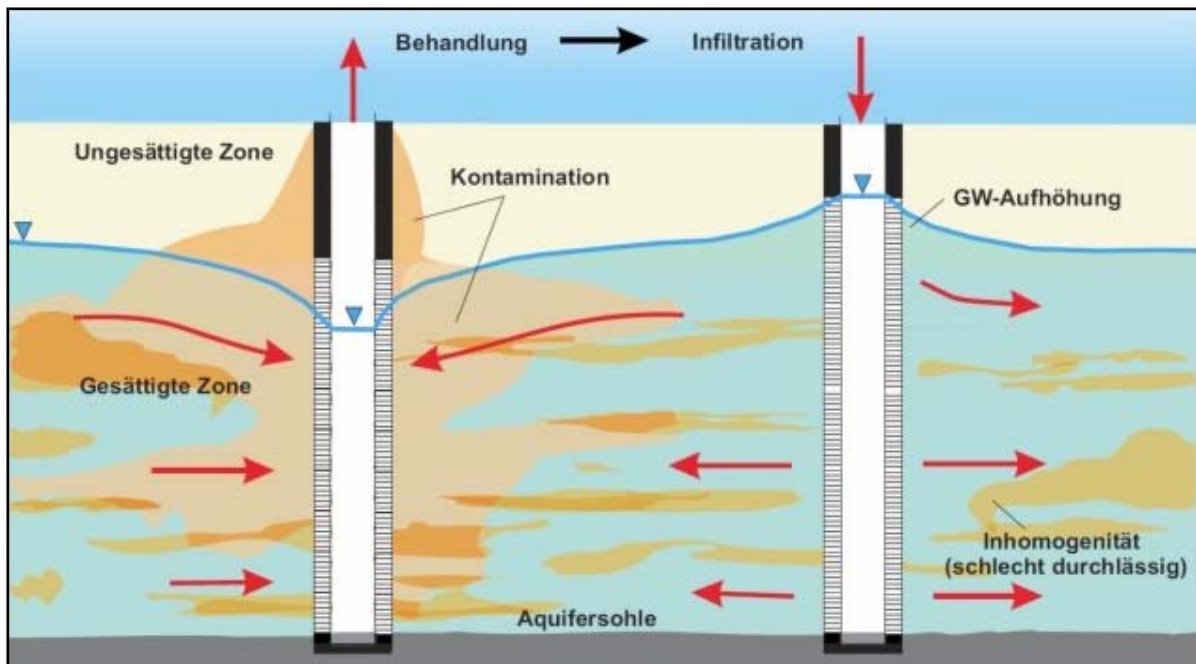
Abbildung 13: Schematischen Funktionsprinzip der Spülung in der ungesättigten Zone (Quelle: www.ieg-technology.com)
