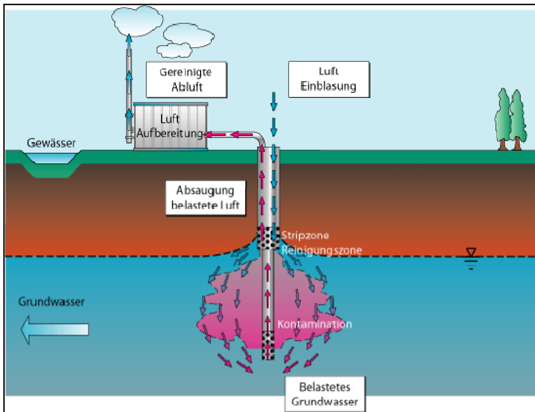
Abbildung 14: Schematischen Funktionsprinzip des Grundwasserzirkulationsbrunnens (Quelle: BAFU)
