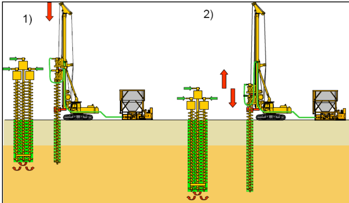
Abbildung 17: schematischen Funktionsprinzip "Mixed in Place" (Quelle: ÖVA, in Vorbereitung, 2009)
