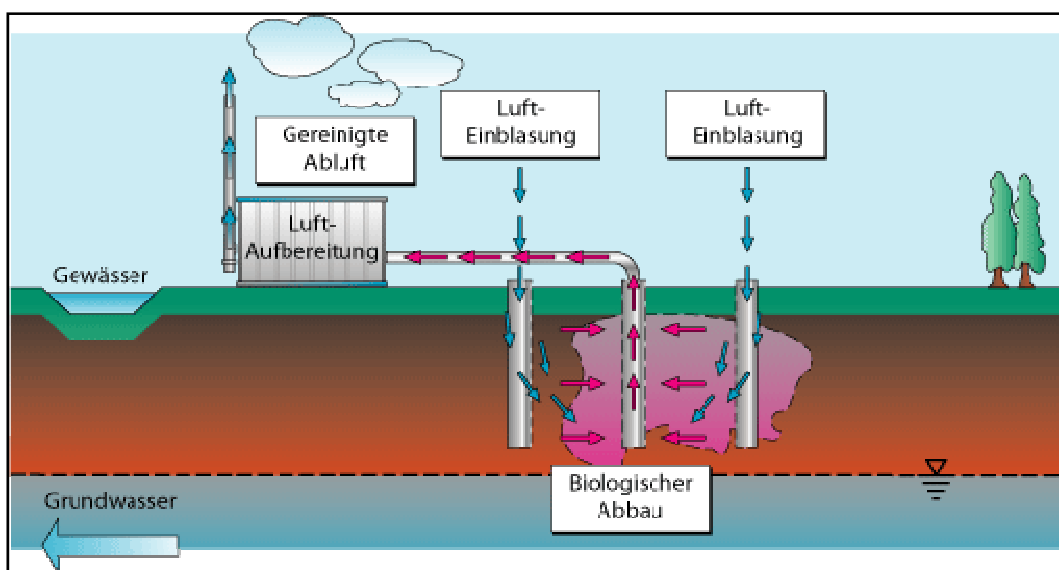
Abbildung 2: Schematisches Funktionsprinzip des Bioventing (Quelle: Bundesamt für Umwelt, BAFU)
