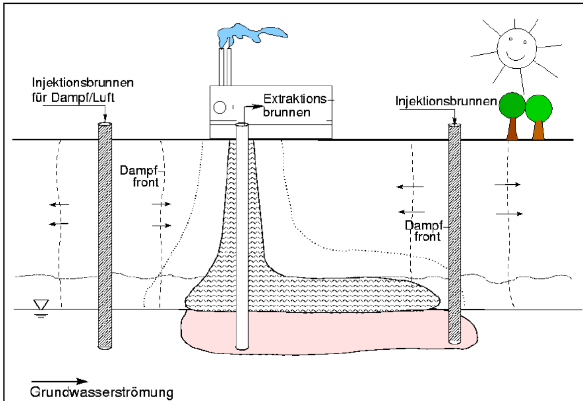
Abbildung 7: In-situ-Dampf-Luft-Injektion (Quelle: Universität Stuttgart)
