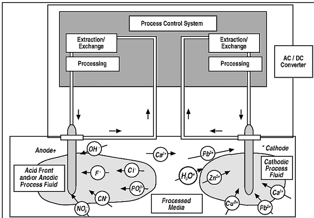
Abbildung 11: Prinzipskizze einer Elektrokinetischen Separation (Quelle: US-EPA)
