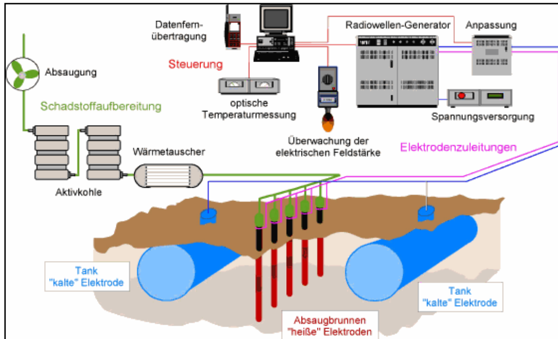
Abbildung 9: Radiofrequenz(RF)-Bodenerwärmung (Quelle: UFZ)
