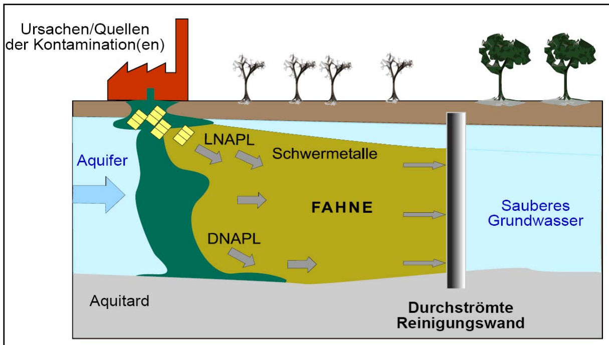
Abbildung 15: Prinzipskizze einer Reaktiven Wand (Quelle: RUBIN 2006)
