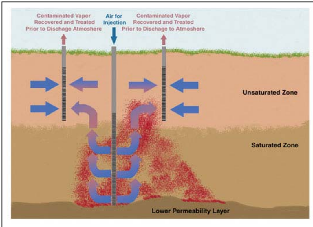
Abbildung 12: Vereinfachtes Schematisches Funktionsprinzip des Air Sparging (Quelle: US-EPA)
