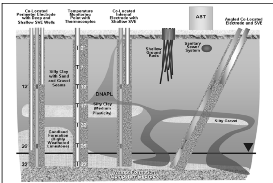
Abbildung 10: Elektrisches Widerstands-Heizen (Quelle: TRS Group)
