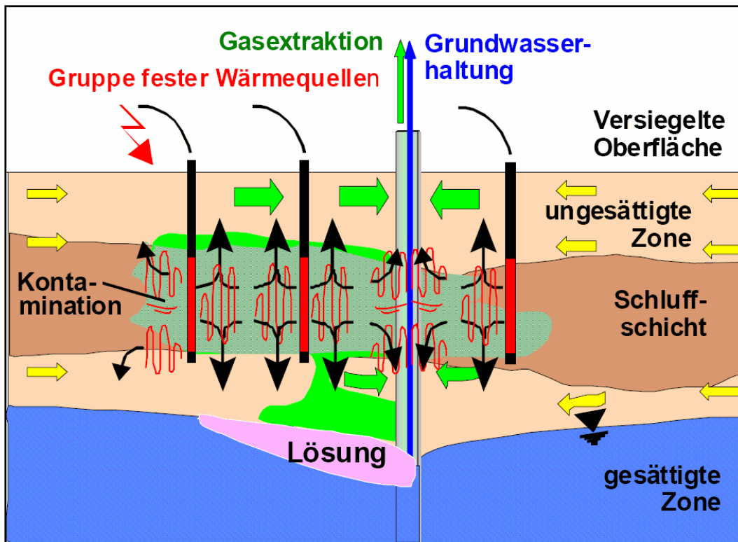
Abbildung 8: Prinzip einer Festen Wärmequelle (Quelle: Universität Stuttgart)
