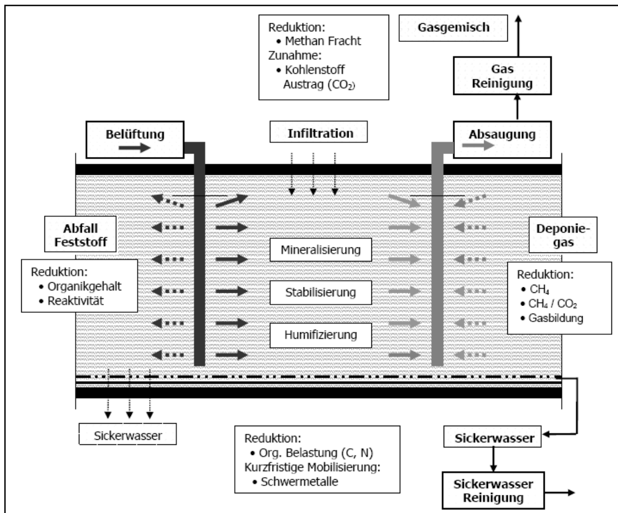
Abbildung 4: Prinzip der In-situ-Aerobisierung (Quelle: Interland 2006)
