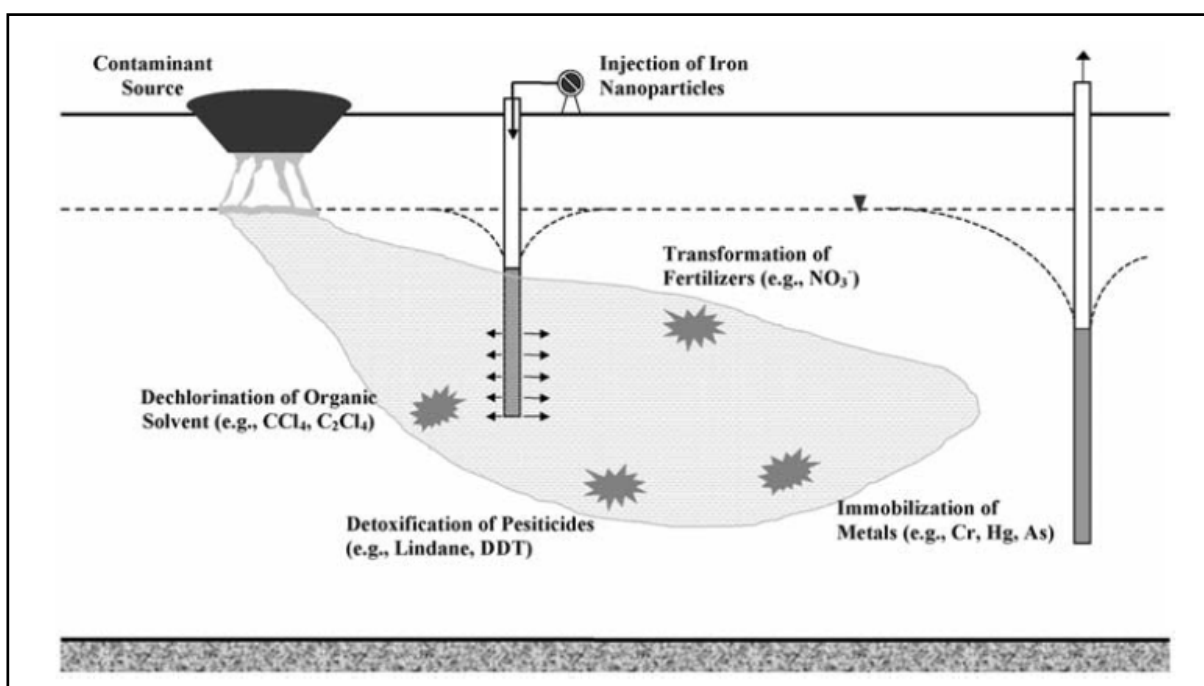
Abbildung 6: Prinzip zur Einbringung von NanoEisen (Quelle: Lehigh University)
