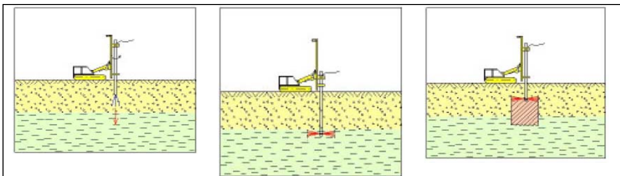
Abbildung 16: schematischen Funktionsprinzip "Düsenstrahlverfahren" (Quelle: Quelle: ÖVA, in Vorbereitung, 2009)
