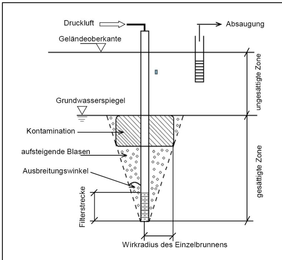
Abbildung 3: Vereinfachtes Schematisches Funktionsprinzip des Biosparging (Quelle: Interland 2006)
